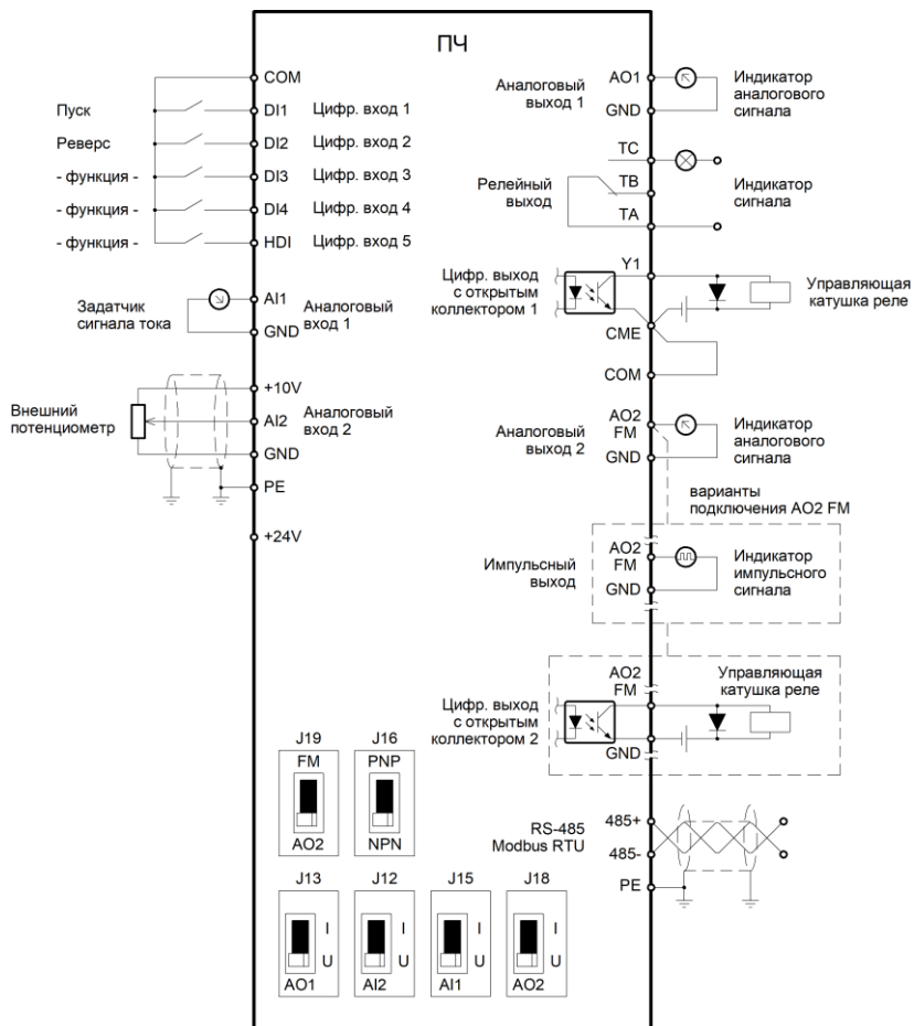
Рисунок 3.10 – Схема подключения управляющих клемм серии NCi для моделей от 37 кВт
