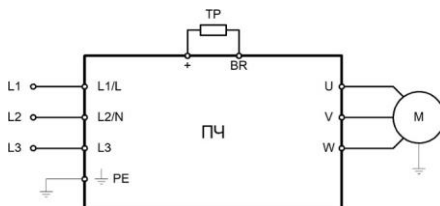
Рисунок 3.4 – Схема силовых подключений для моделей NCI-GY/PY-4B до 30 кВт
