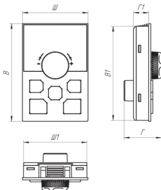
Рисунок 5.2 – Выносная панель управления NCI-KP
