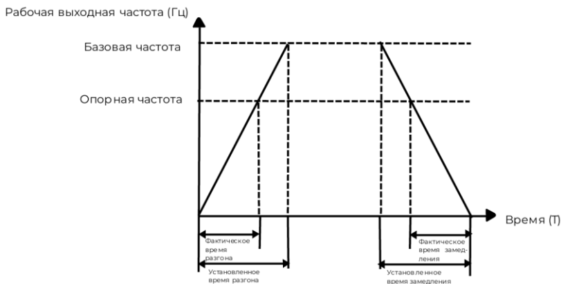
Рисунок 6.3 – Время разгона/замедления
