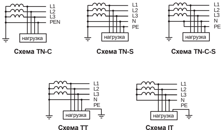
Рисунок 3.12 – Типы систем заземления
