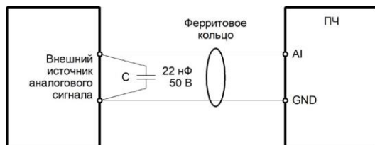
Рисунок 3.16 – Схема подключения проводов к аналоговому входу (при воздействии сильных помех)
