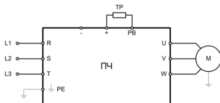
Рисунок 3.5 – Схема силовых подключений для моделей NCI-GY/PY-4B от 37 кВт
