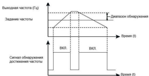
Рисунок 6.17 – Диапазон достижения максимальной частоты
