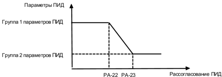
Рисунок 6.21 – Переключение параметров ПИД
