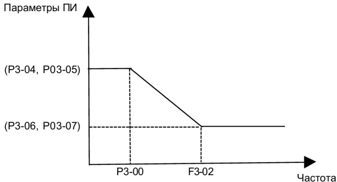
Рисунок 6.8 – Зависимость параметров ПИ от частоты
