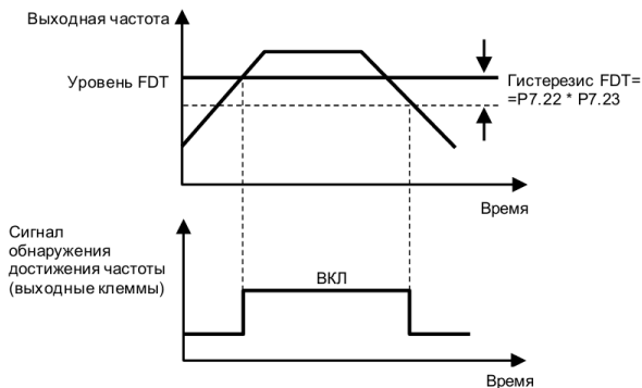
Рисунок 6.16 – Значение обнаружения выходной частоты
