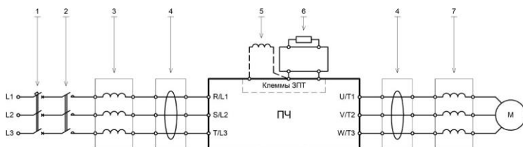
Рисунок 3.6 – Схема подключения дополнительного оборудования
