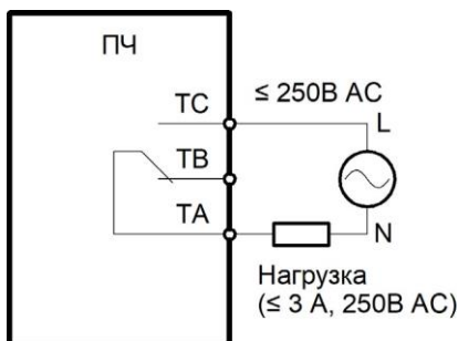
Рисунок 3.17 – Схема подключения нагрузки переменного тока к релейному выходу
