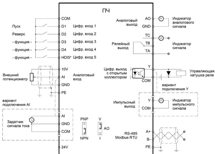
Рисунок 3.9 – Схема подключения управляющих клемм серии NCI для моделей до 30 кВт
