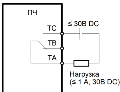
Рисунок 3.18 – Схема подключения нагрузки постоянного тока к релейному выходу
