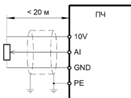
Рисунок 3.15 – Схема подключения проводов к аналоговому входу (общий случай)
