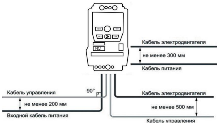
Рисунок 3.13 – Графическое представление расстояний между кабелями
