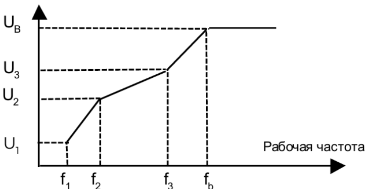
Рисунок 6.7 – Ломаная характеристика U/f
