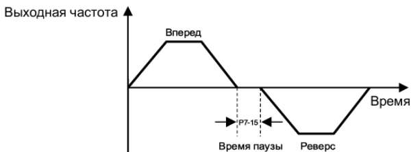
Рисунок 6.15 – Время паузы при смене направления вращения
